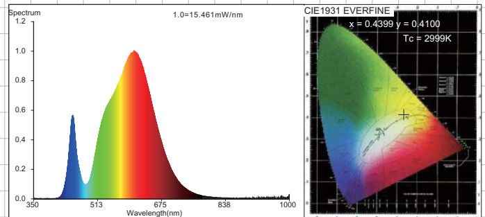
B5 T3 2U E27 10W 3000K
