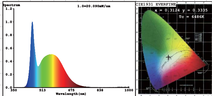
B5 T3 2U E27 8W 6400K
