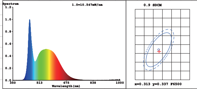
B5 T3 2U E14/E27 4W 6400K
