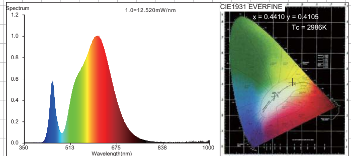
B5 T3 2U E27 8W 3000K
