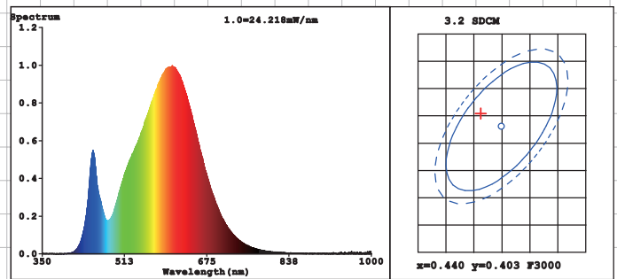
B5 T3 4U E27 15W 3000K
