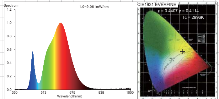
B5 T3 2U E14/E27 6W 3000K
