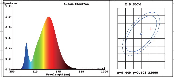
B5 T3 2U E14/E27 4W 3000K
