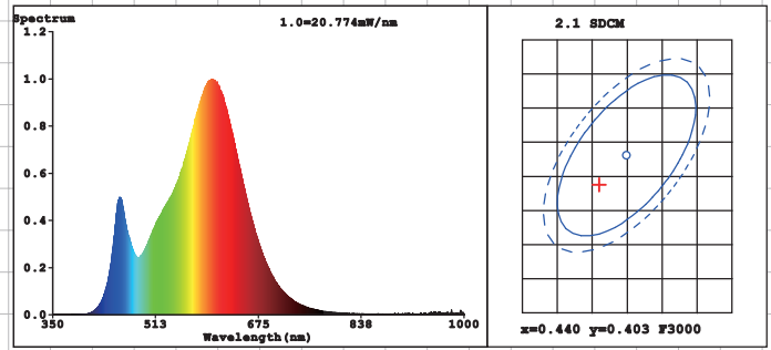
B5 T3 3U E27 12W 3000K
