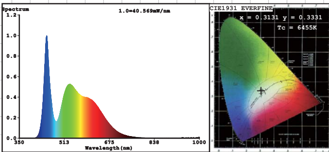
B5 T3 4U E27 15W 6400K
