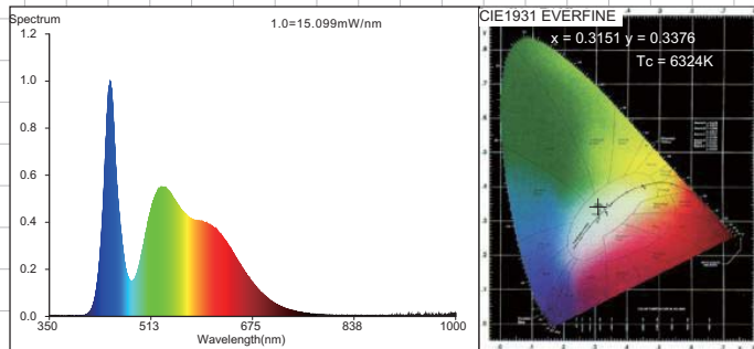
B5 T3 2U E14/E27 6W 6400K
