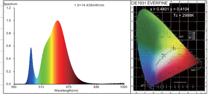
B5 T3 3U E27 9W 3000K
