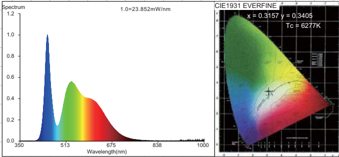
B5 T3 3U E27 9W 6400K
