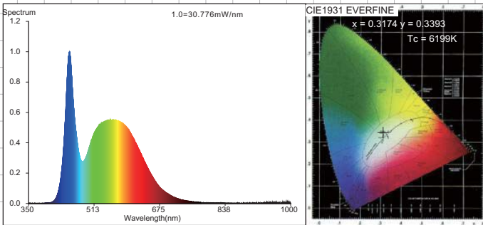
B5 T3 3U E27 12W 6400K
